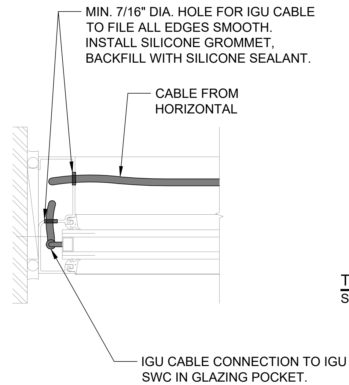
DETAIL 4 LEFT JAMB
